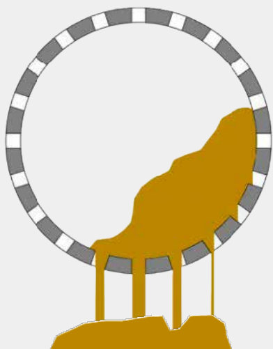
Siebtrommel mit großer Maschenweite & hoher Blechstärke liefert im Gegenzug einen geringeren Materialdurchsatz bei höherer Lebensdauer
